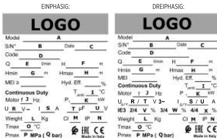
Abb. 2: Typenschild der Elektropumpe
